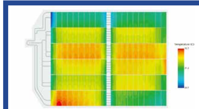
直冷板仿真
