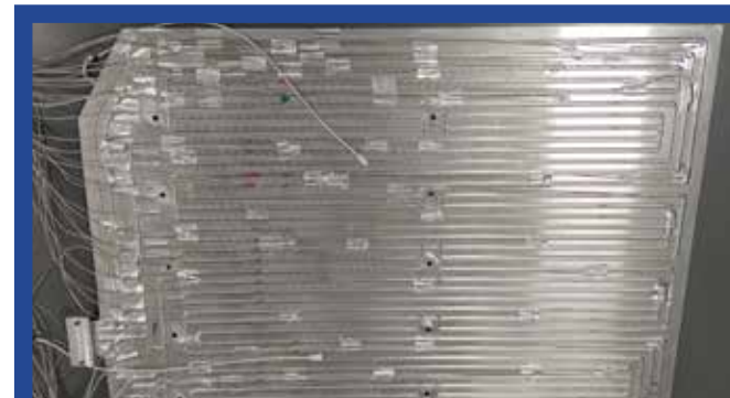
直冷板均温试验
